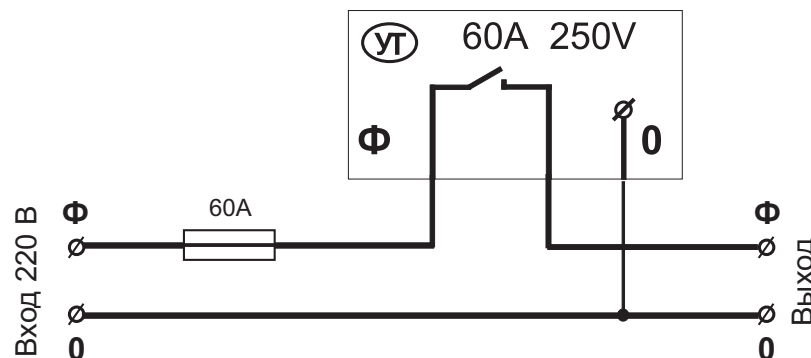
Рис.1 Схема подключения прибора.
