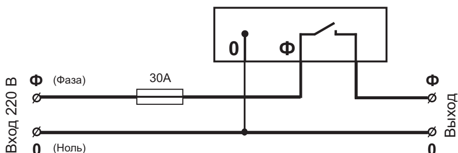
Рис.1 Схема подключения прибора. В качестве предохранителя может быть токовый автомат соответствующего номинала.
