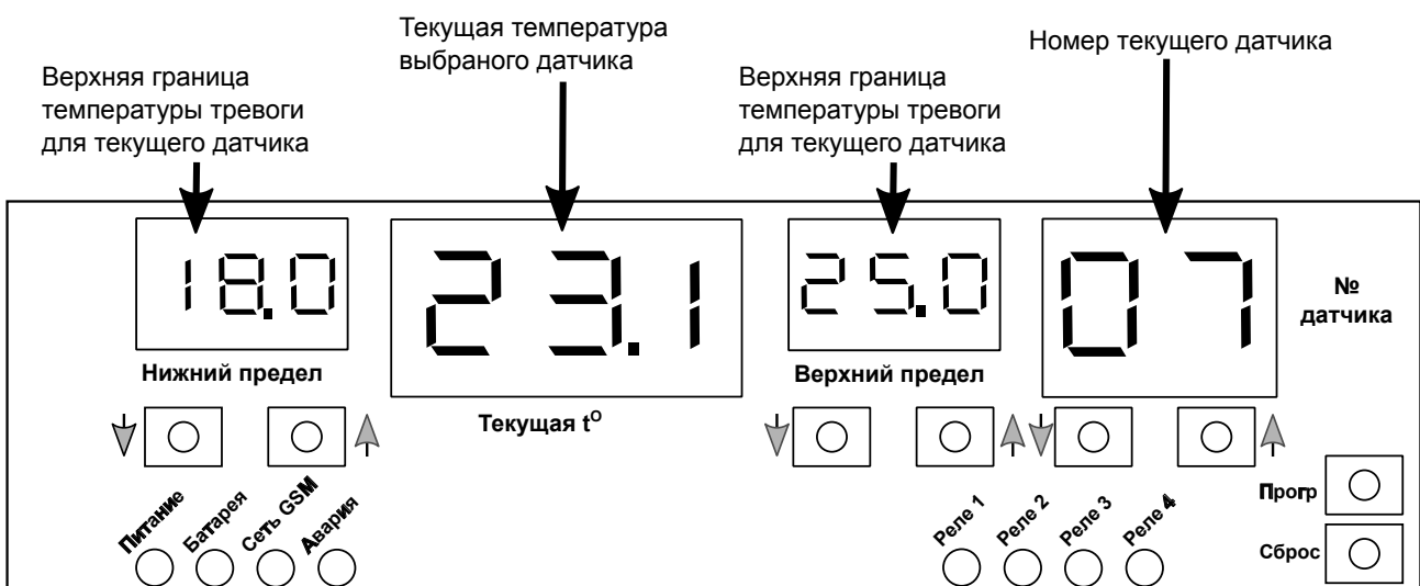
Рис. 9. Основной экран
