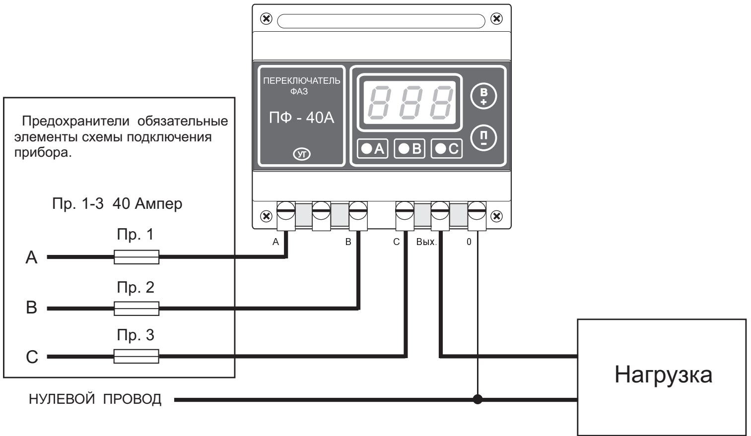
Схема подключения прибора к 3х фазной электросети.
