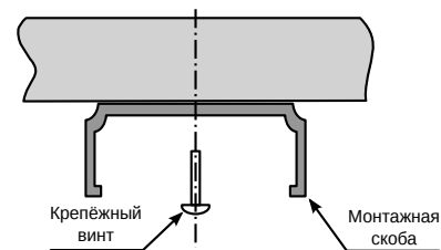
Крепление к поверхности
