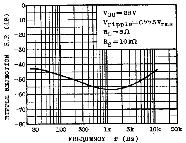
R.R - f
