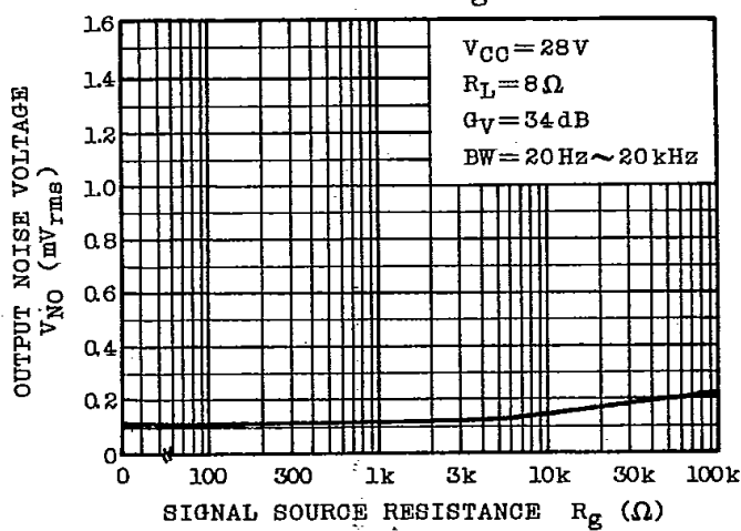
V_{NO} - R_g
