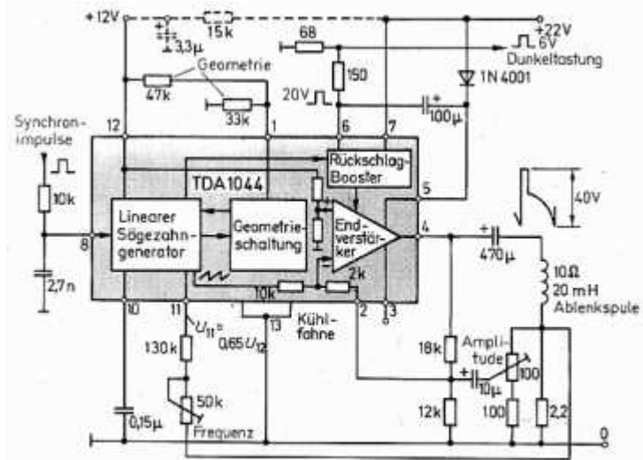
Bild 6.45 Vertikaleblenkung eines 110°-Schwarz-Weiß-Fernsehempfängers mit dem IC: TDA 1044 (ITT)
