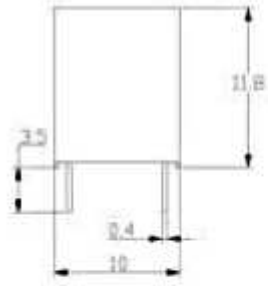
安装图
