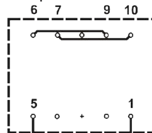
Параллельное соединение вторичных обмоток
