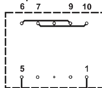
Параллельное соединение вторичных обмоток
